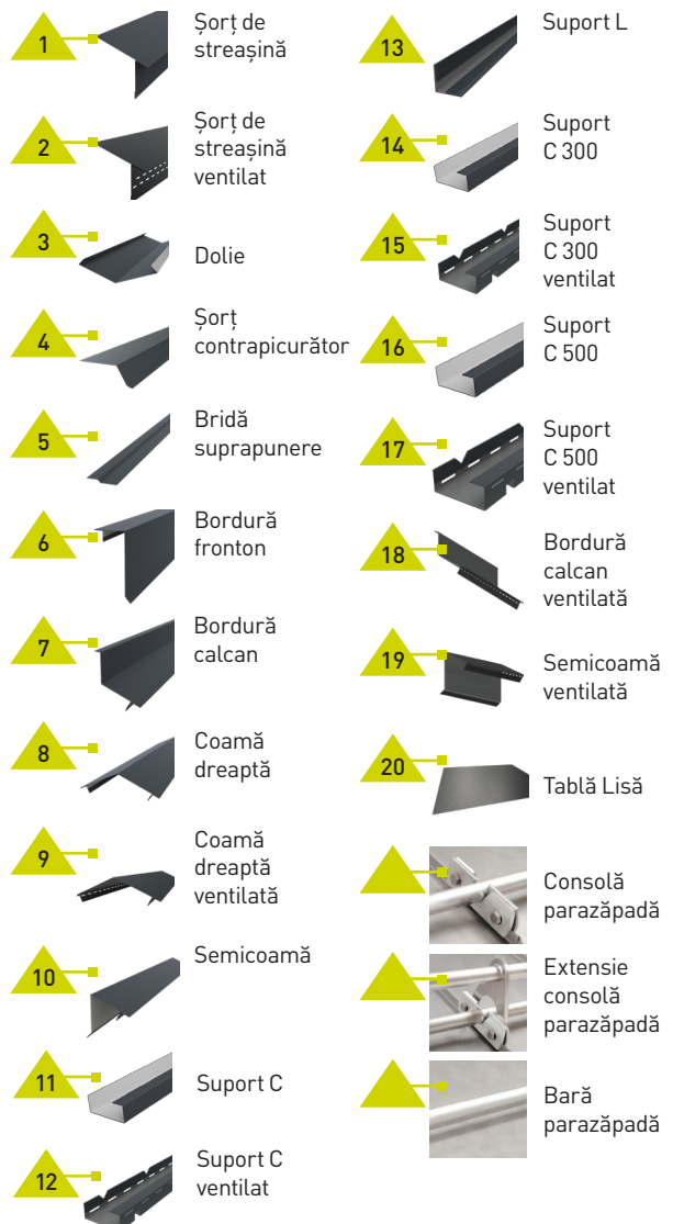
Piese de finisaj TABLĂ PREFĂLȚUITĂ
